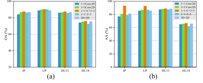
Fig. 11. Ablation study on the SSFE. (a) OA. (b) AA.
